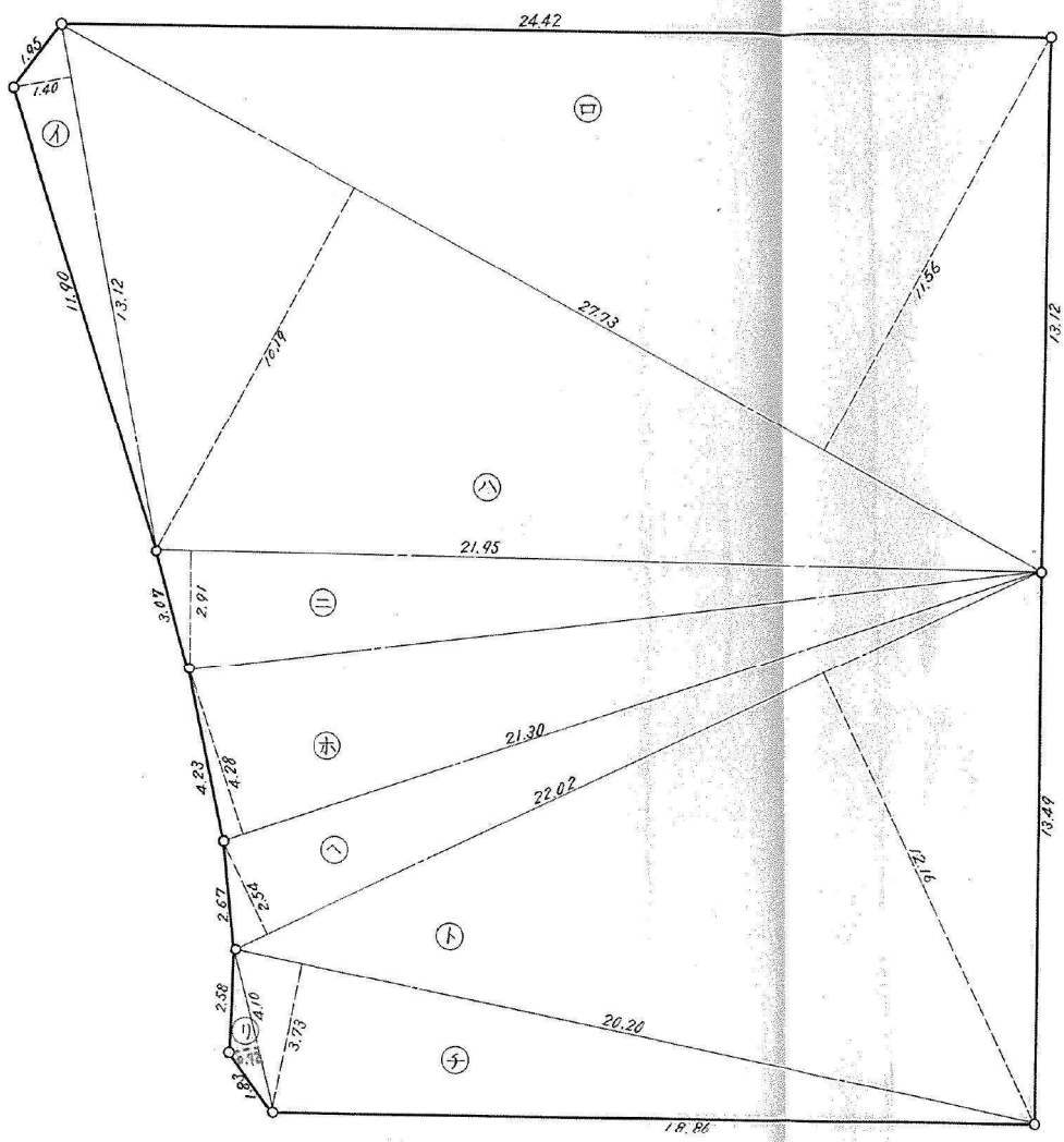
F-5 ① 丈量図 S = 1/300
